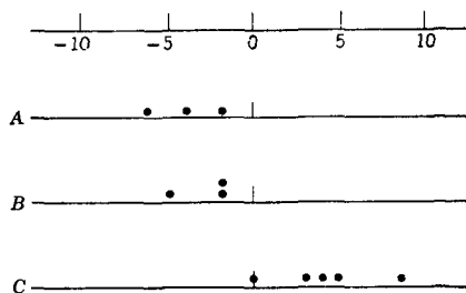
Рис. 3.6. График остатков, указывающий из блоковые эффекты, не связанные с подобранной моделью
