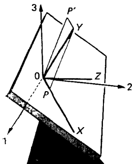
Рис. 4.3. Геометрическая интерпретация регрессии Y на X
