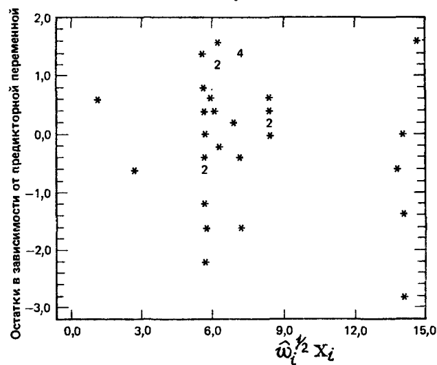
Рис. 2.4. Графики остатков при взвешенном методе наименьших квадратов
