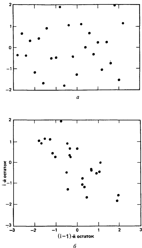
Рис. 3.8. (а) Серия остатков, проявляющих локально отрицательную сериальную корреляцию, обусловленную, быть может, транспортным запаздыванием. (б) График сериальной корреляции с единичным сдвигом для тех же данных
