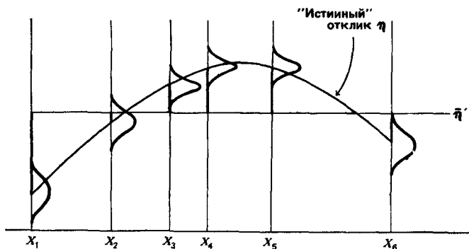
Рис. 2B.1. Отклонения «истинных» величин \eta относительно их среднего по сравнению с размахами оценок \hat{Y}_i - \tilde{Y}_i для одной переменной X
