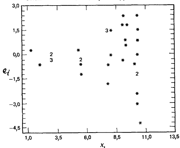
Остатки в зависимости от предикторной переменной
