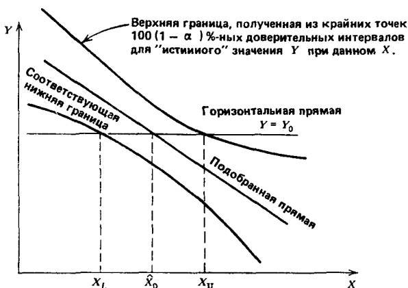
Рис. 1.11. Обратная регрессия: оценивание X по \hat{X}_0 для данного значения Y_0 и получения 100(1-α) %-ных «фидуциальных интервалов» для X
