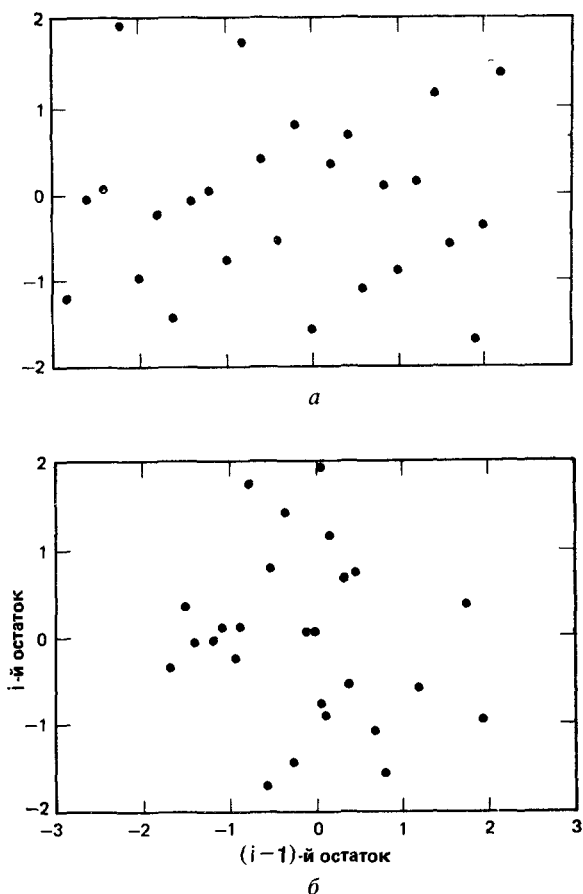
Рис. 3.9. (а) Серия некоррелированных остатков. (б) График сериальной корреляции с единичным сдвигом для тех же данных
